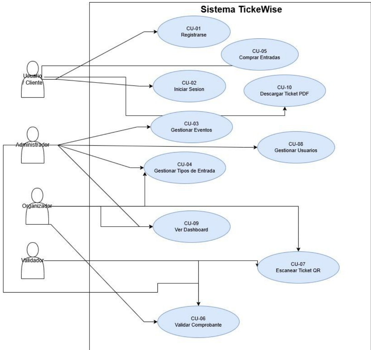
Figura 3. Caso de Uso del Sistema Ticketwase
