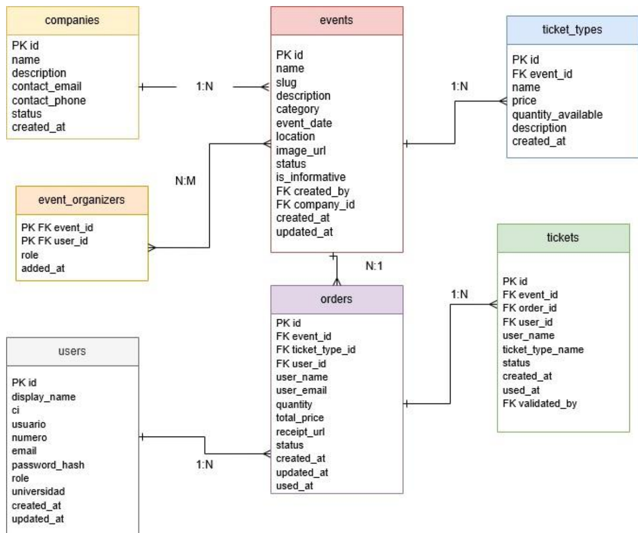
Figura 2. Diagrama Entidad Relacion del Sistema
